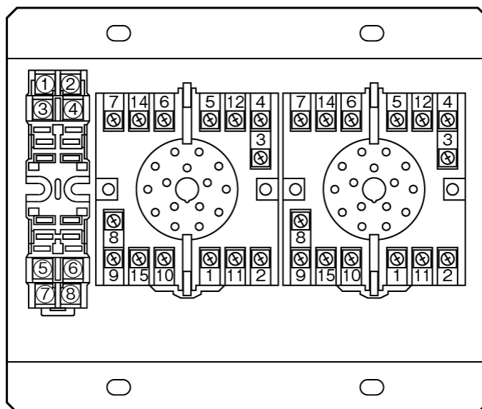
図1. 2 端子台全体図
