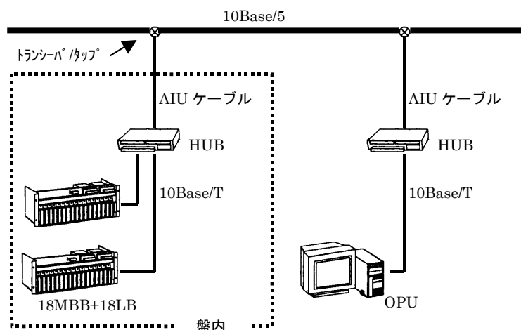
図 8. 1 L-Bus システム構成図
