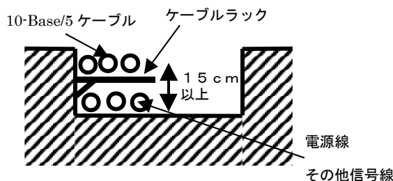
図 8. 3 ピットのケーブルラック
