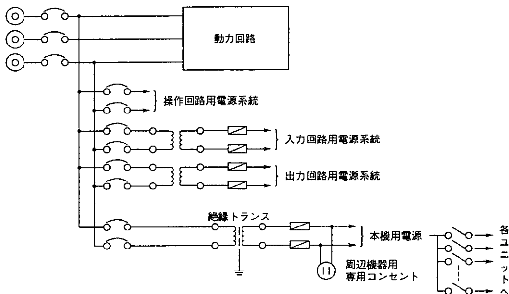
図3. 1 電源系統図
