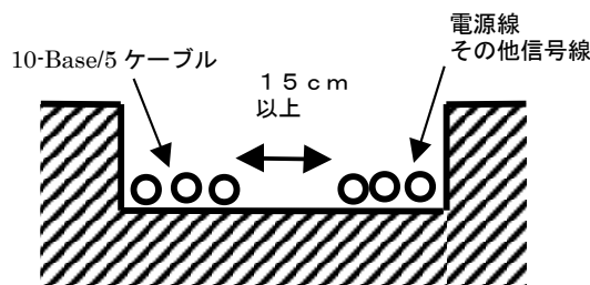
図 8. 4 ピット、フリーアクセス床下のケーブル間隔
