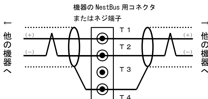
図 6. 2 NestBus ケーブルの接続
