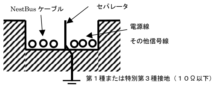
図 6. 4 ダクト、ピットのセパレータ
