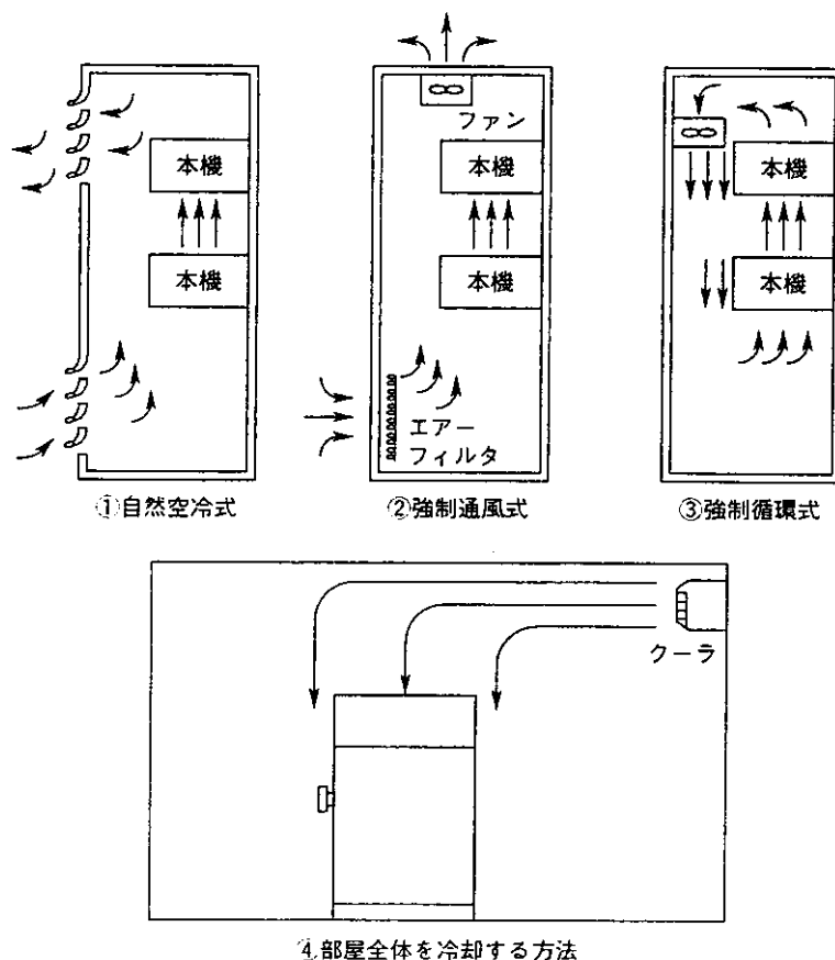
図2. 1 代表的な冷却方式
