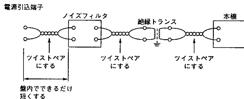
図 2. 2 電源回路のノイズ対策例
