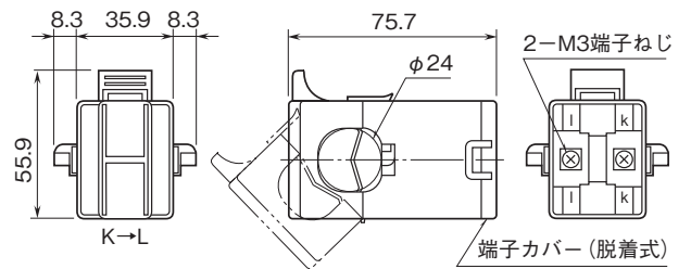
■クランプ式センサ:CLSB-40
