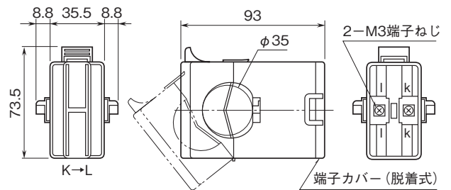
■クランプ式センサ:CLSB-60
