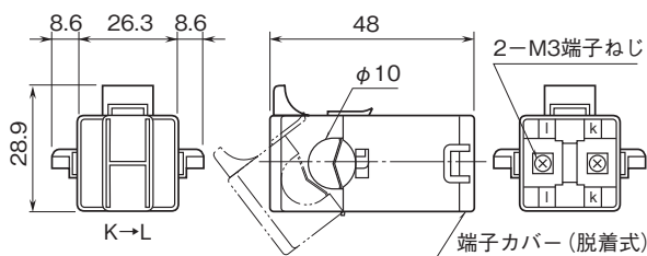
■クランプ式センサ:CLSB-05
