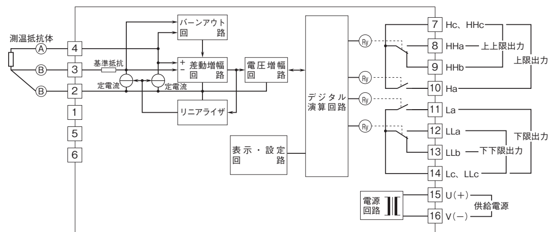
■48NDR-4 (4点警報/4接点出力)
