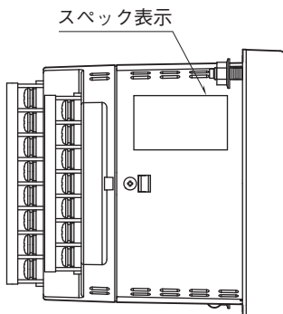
■左側面図
