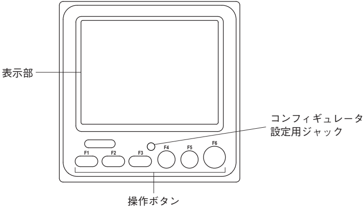
■前面図
