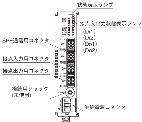
■前面図
