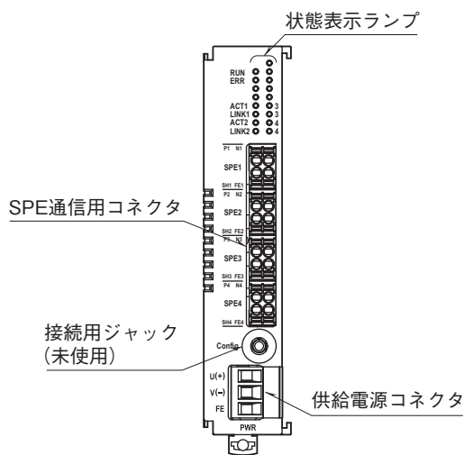
■前面図
