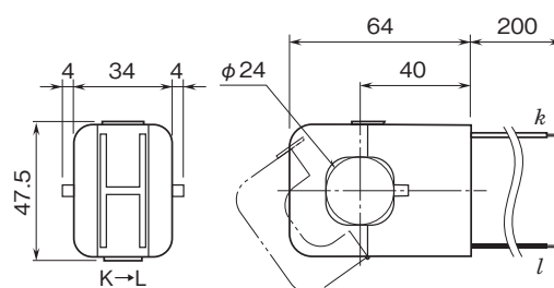
■クランプ式センサ:CLSA-30
