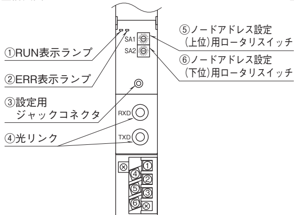
■前面図
