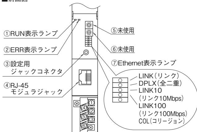
■前面図
