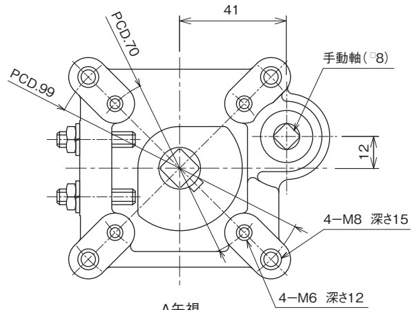
A矢視
