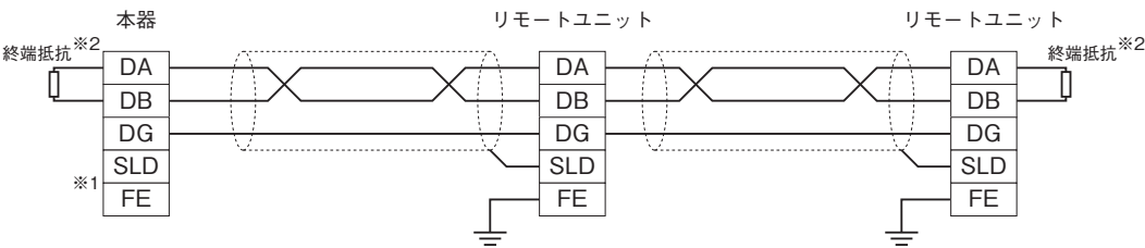
■スレーブ機器との配線
