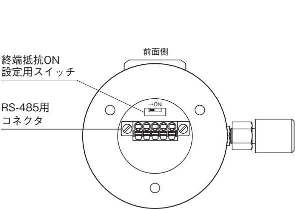
■底面図
