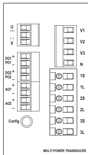
■外部インタフェースコード：6、7
