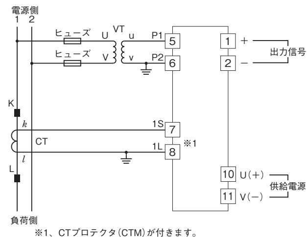
单相2線式
