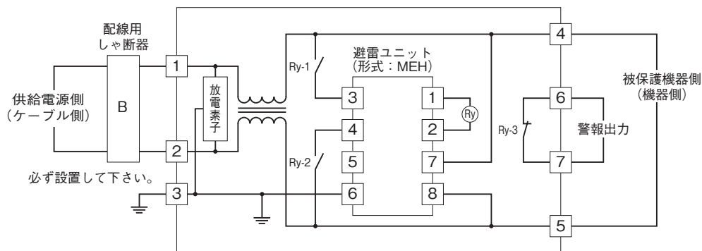
・避雷ユニット (形式:MEH) ブロック図
