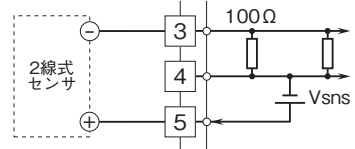
■2線式電流パルス入力
