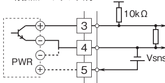
■オープンコレクタまたは有接点スイッチ入力
