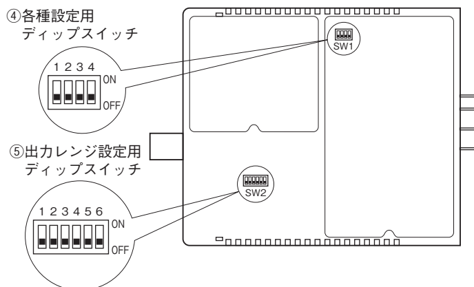
■右側面図
