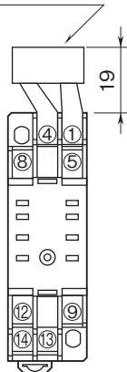
入力抵抗器 (REM2)
