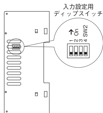
■右側面図
