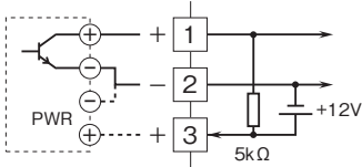
入力部接続例
