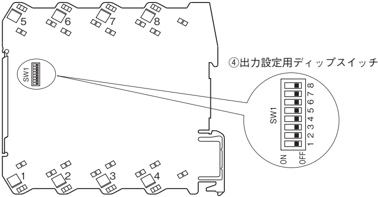
■側面図
