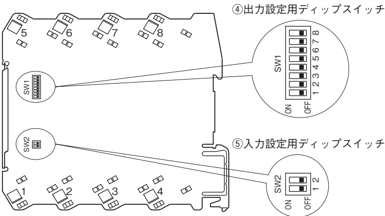
■側面図
