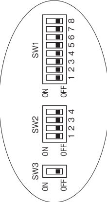
④各種設定用ディップスイッチ
