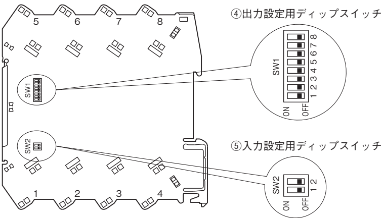
■側面図
