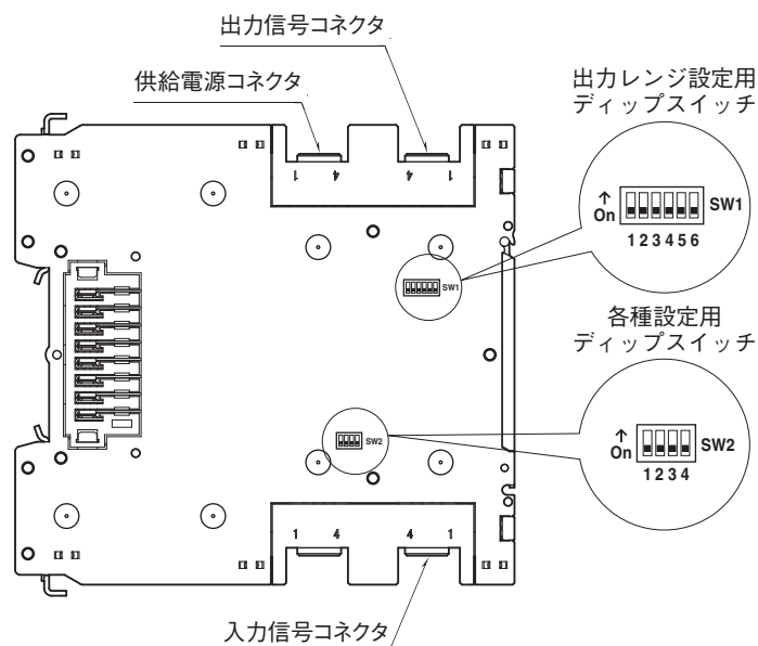
■左側面図
