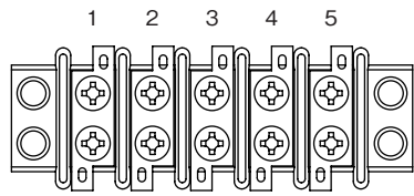
■内部端子台配線図
