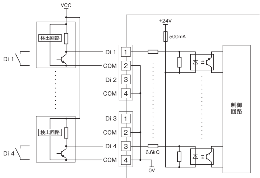
■入力回路
