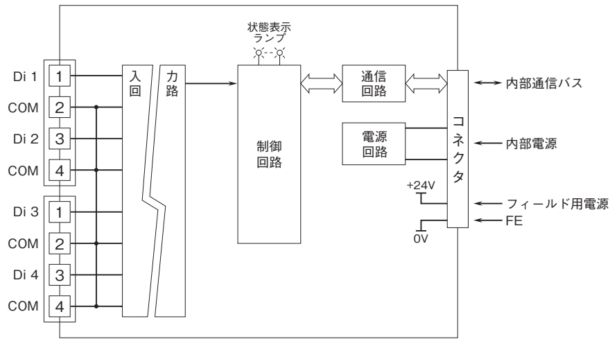
■入力回路
