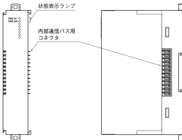
■前面図
