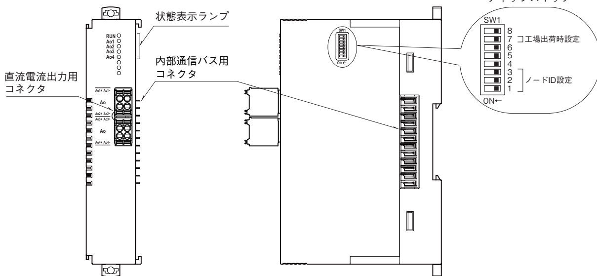
■前面図
