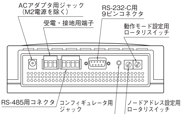
■背面図
