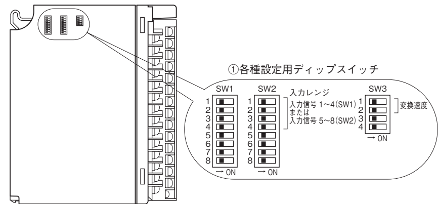
■側面図
