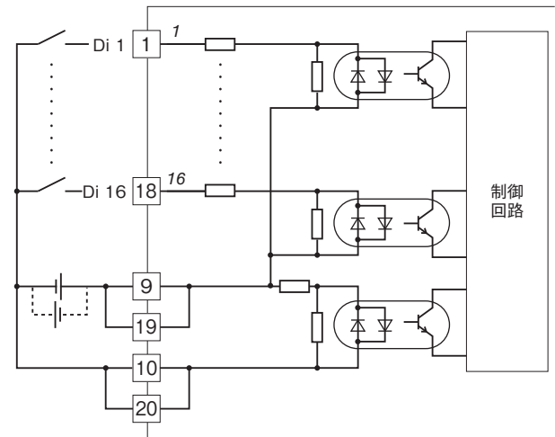
■入力回路
