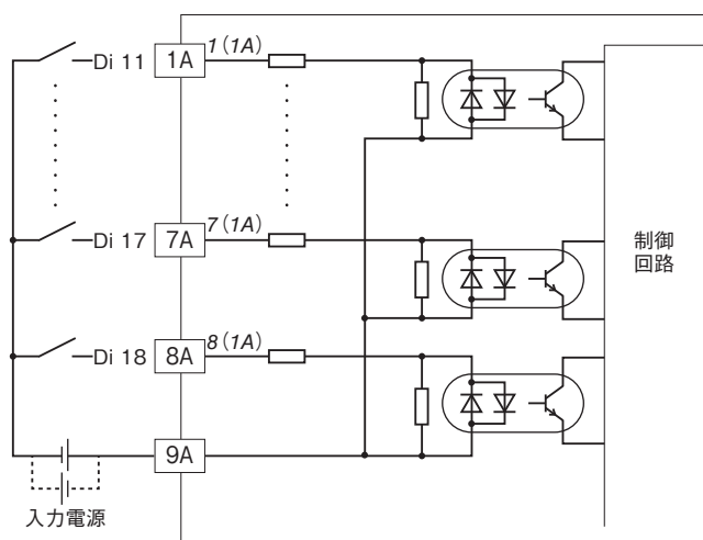
■入力回路
