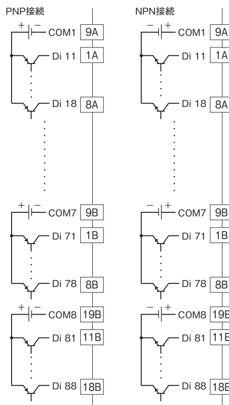
■入力部接続例
