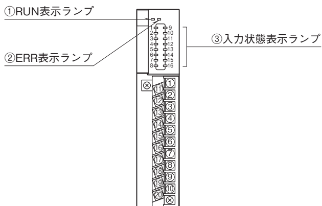
■前面図
