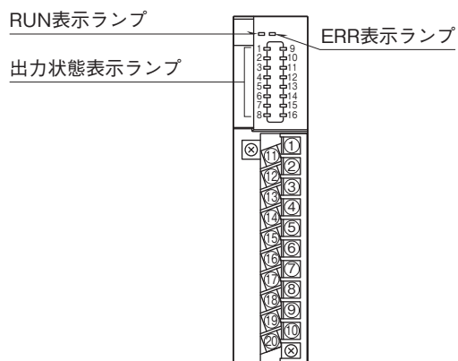
■前面図
