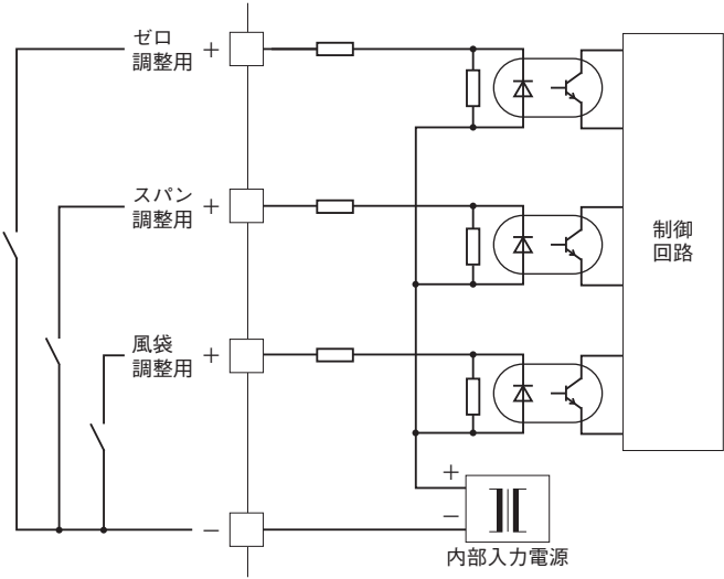
■接点入力回路
