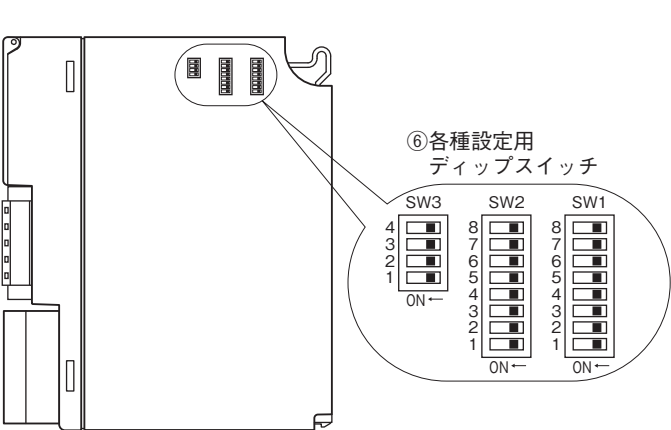
■側面図
