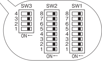
⑥各種設定用 ディップスイッチ
