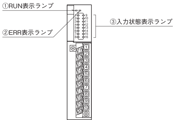
■前面図
