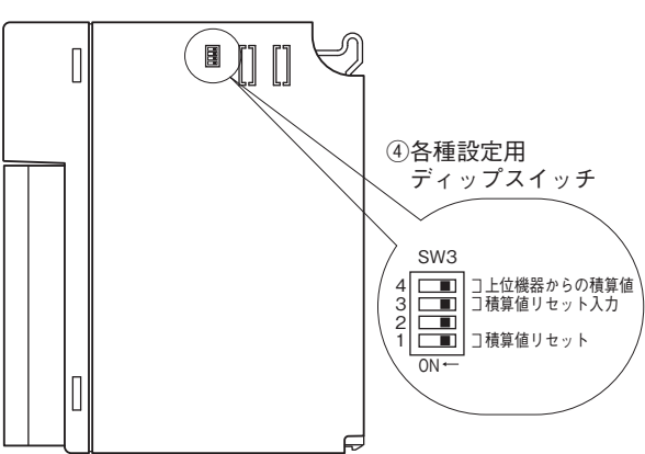
■側面図
