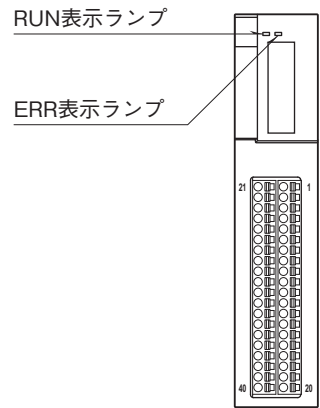
■前面図
