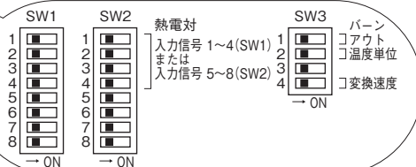
①各種設定用ディップスイッチ
