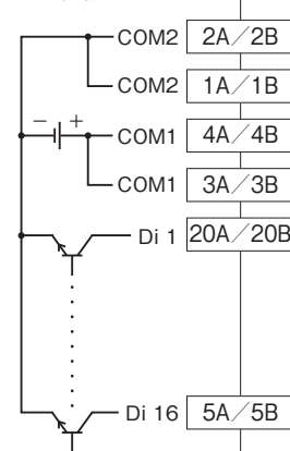
NPN接続
