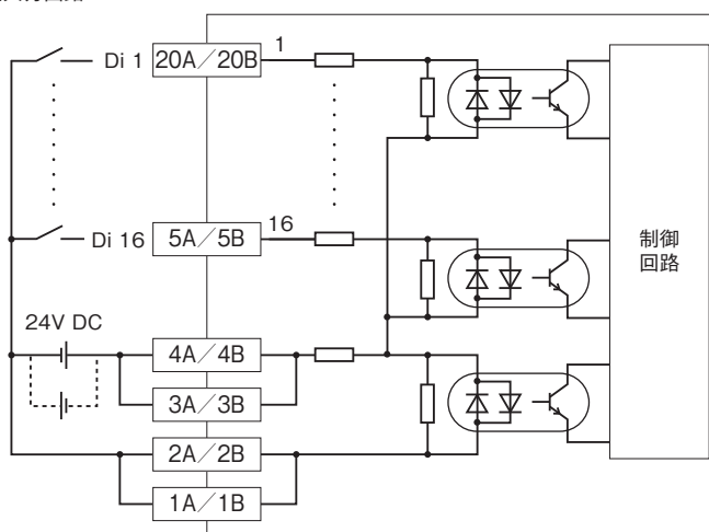
■入力回路
