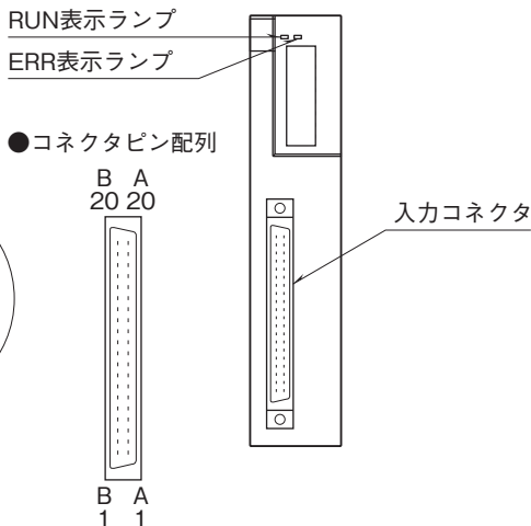
■前面図
