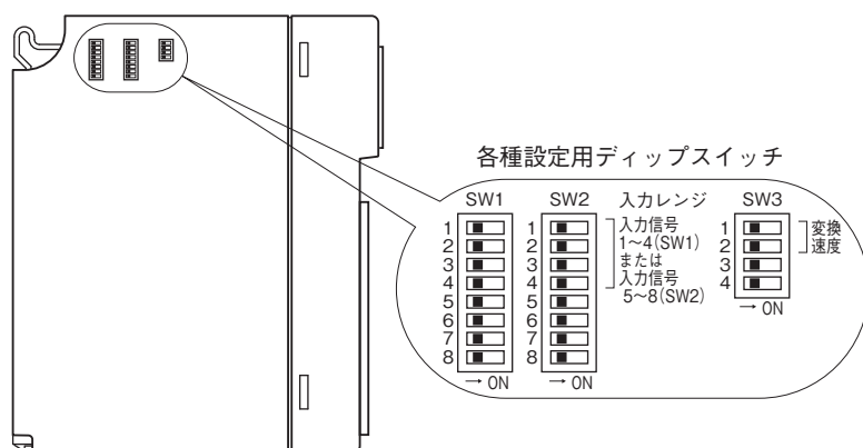
■側面図
