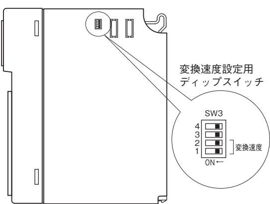
■側面図
