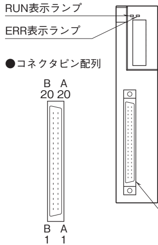
■前面図
