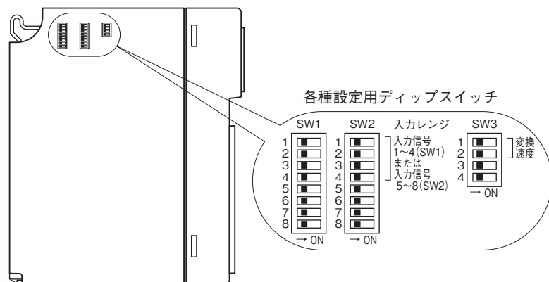
■側面図
