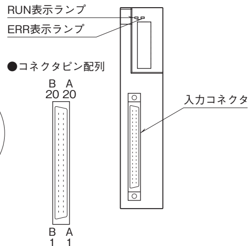
■前面図
