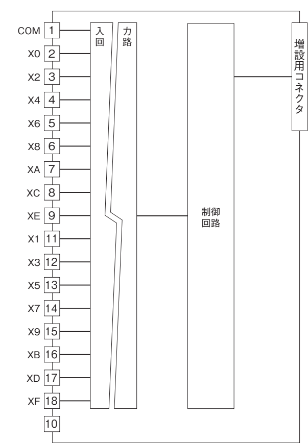
■入力回路
