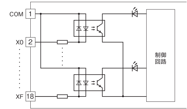
■入力回路
